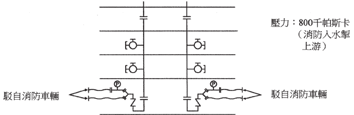
圖 3.2 裝置2條或以上上水喉管的其他建築物（1 800 公升／分鐘）
