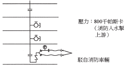
圖 3.2 裝置2條或以上上水喉管的其他建築物（1 800 公升／分鐘）
