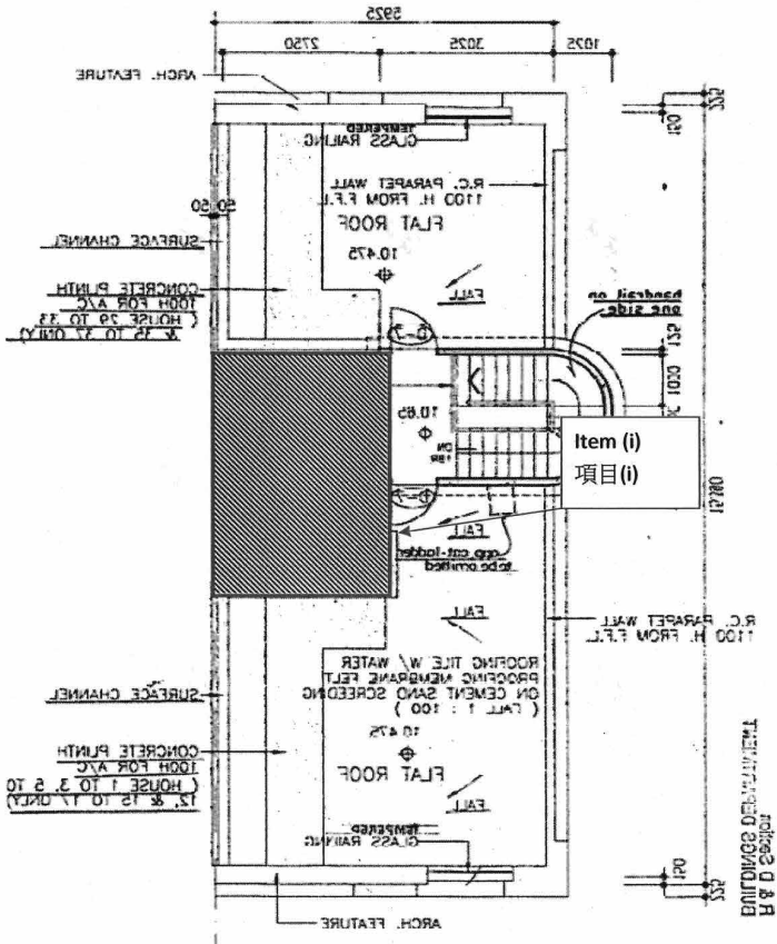
R/F Plan 天台平面圖
