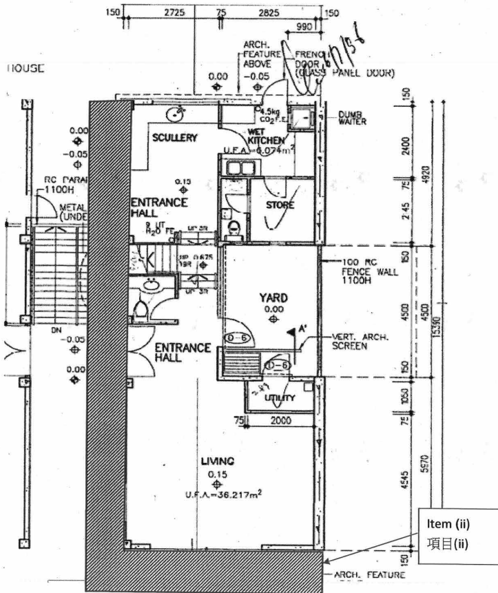
G/F Plan 地面平面圖
