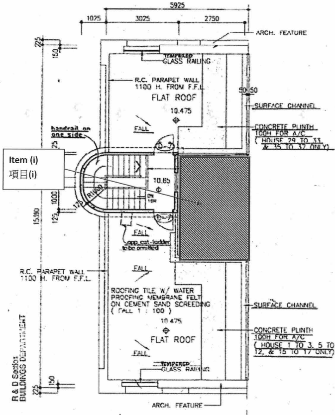
R/F Plan 天台平面圖
